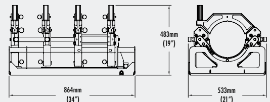
DYNAMC 250 AUTO
